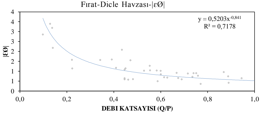
Şekil 4.5-3: F-D Havzasında |\varepsilon_0| değerlerinin debi faktörü ile değişim
